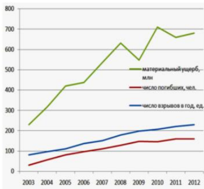
График изменения числа взрывов природного газа в России в жилом секторе в период 2003–2012 гг.
